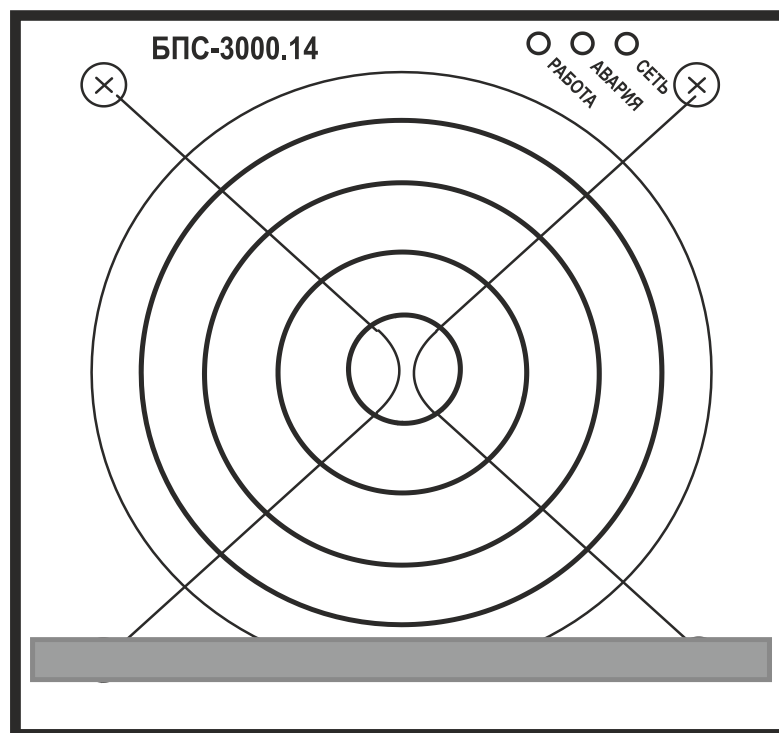
Рис.2. Вид БПС спереди.
