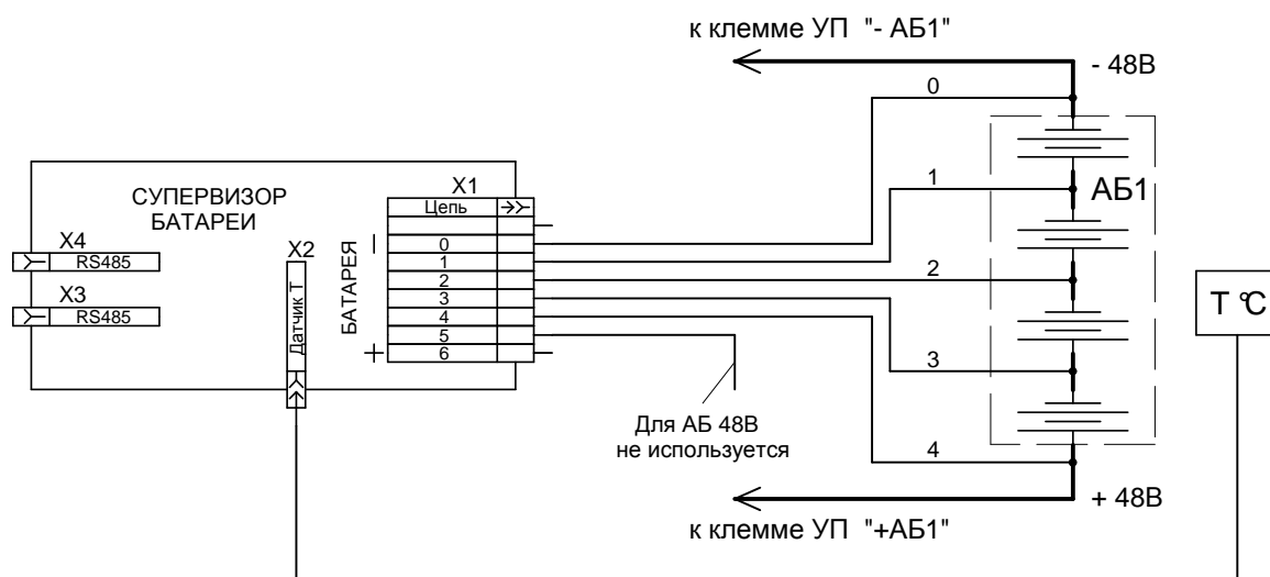
Рисунок 2.1 – Подключение модуля САБ
