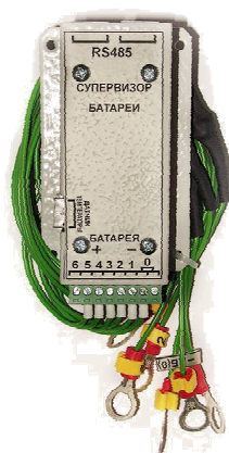
Рисунок 1.6 – Супервизор аккумуляторных батарей
