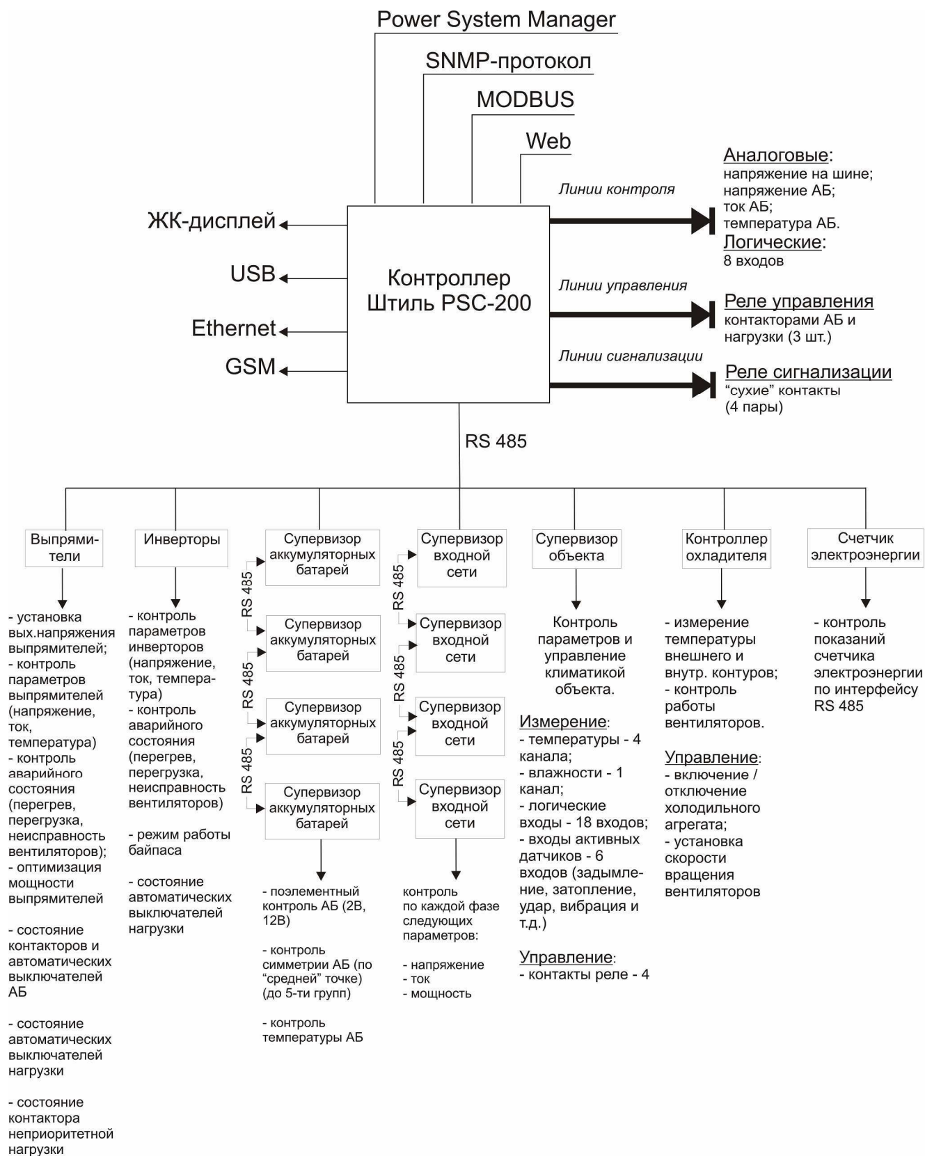
Рисунок 1. 4 - Структура контроллера Штиль PSC-200 (максимальная конфигурация)
