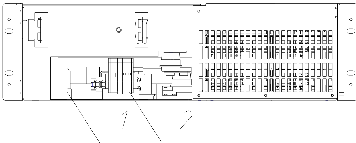
1 – вывод заземления, 2 – выходы подключения СЕТЬ ~220В (N, L1, L2, L3) Рисунок 1.3 – Установка питания постоянного тока Штиль PS48-0080-3U. Вид с тыльной стороны
