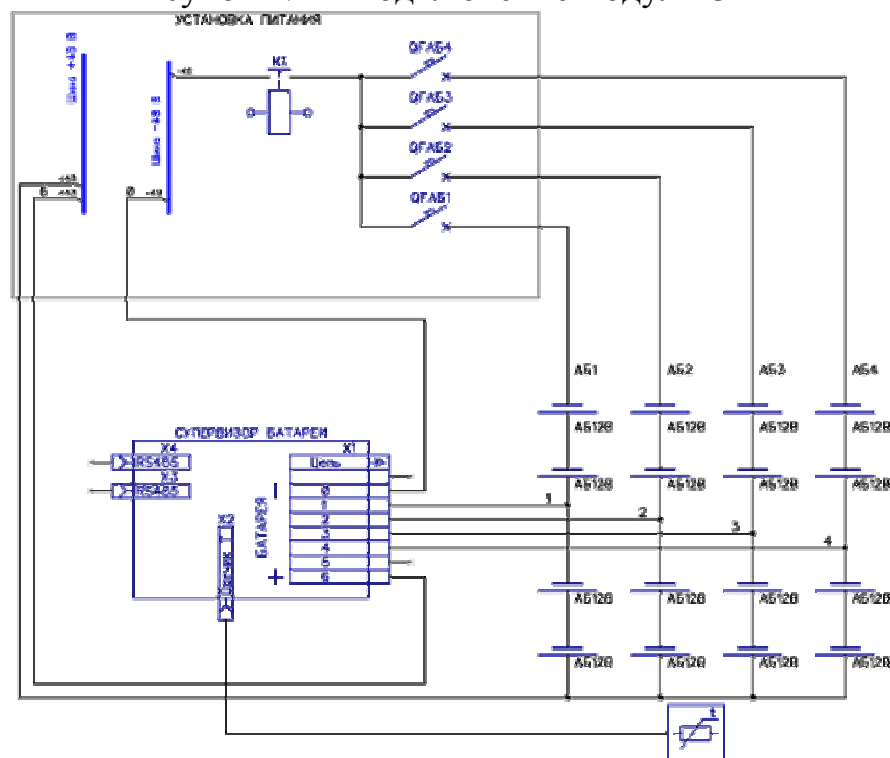
Рисунок 2.2 – Подключение модуля САБ. Контроль симметрии.
