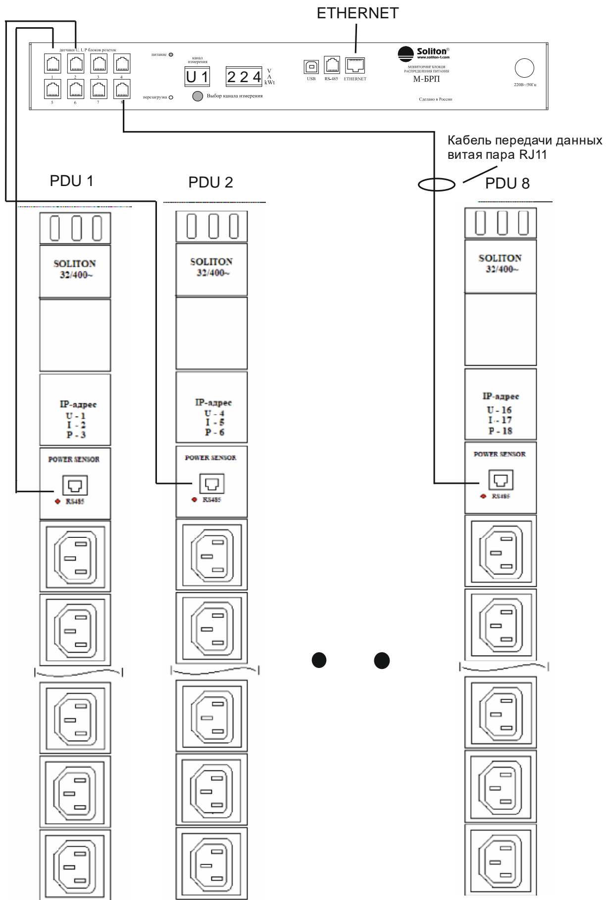
Рис.3 Схема подключения однофазных БРП к системе мониторинга
